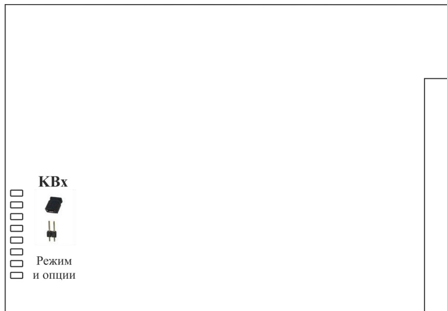
Рисунок 5 – Размещение элементов на верхней плате прибора Тема-А82.22-м51
