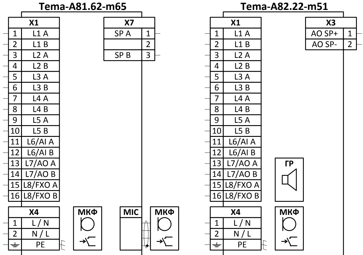
Рисунок 3 – Условное графическое обозначение прибора Тема-А8х.х2
