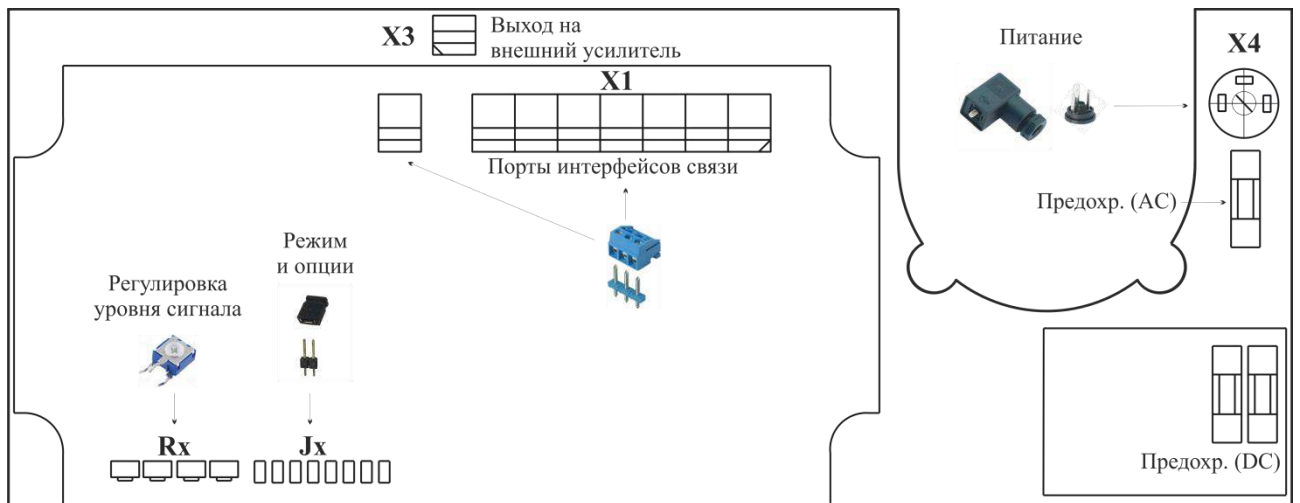
Рисунок 4 – Размещение элементов на нижней плате прибора Тема-А82.22-м51
