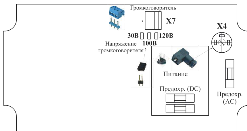
Рисунок 7 – Размещение элементов на нижней плате прибора Тема-А81.62-м65
