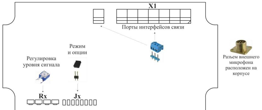
Рисунок 6 – Размещение элементов на верхней плате прибора Тема-А81.62-м65
